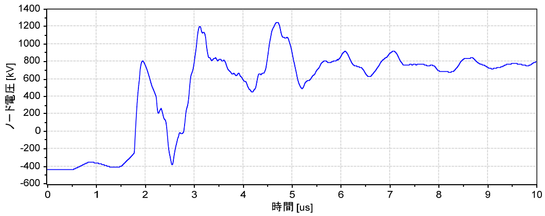
(b) 変電所入口
