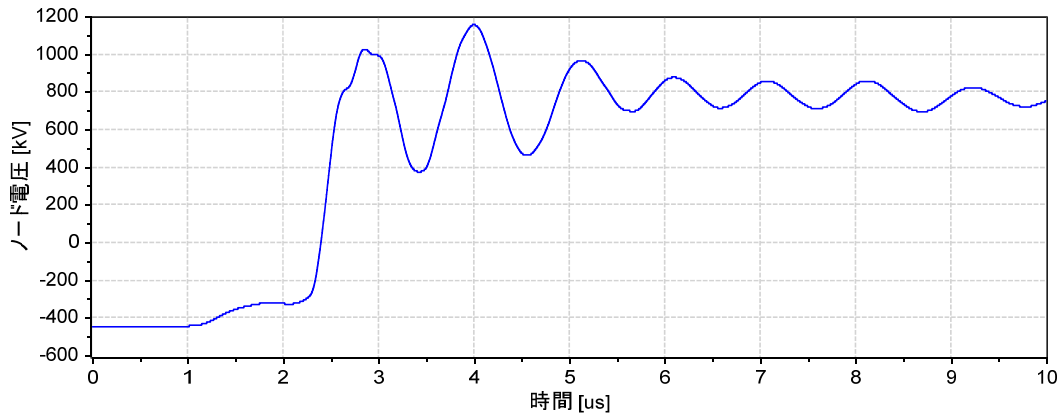
(c) 母線電圧波形 (変圧器端)
