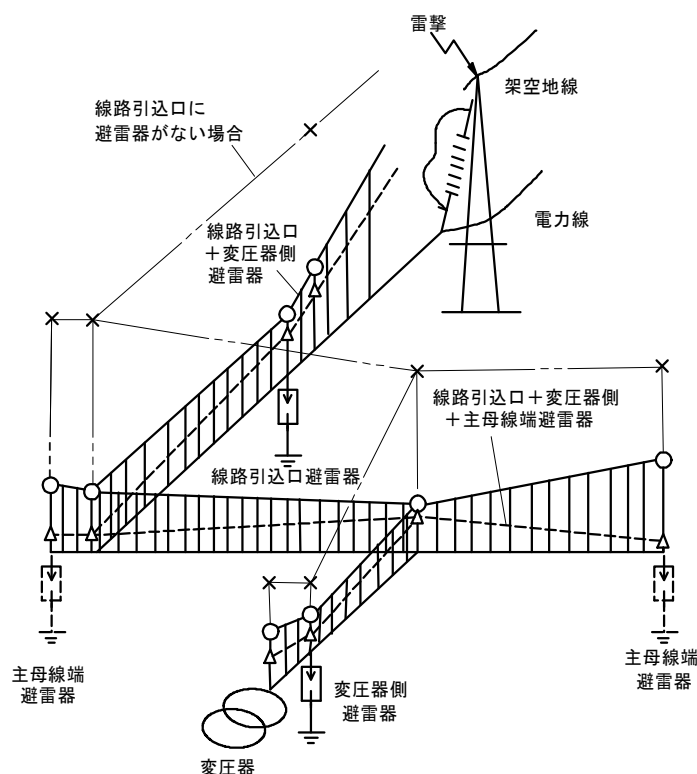
図 1 変電所の雷サージ伝搬の概念図
