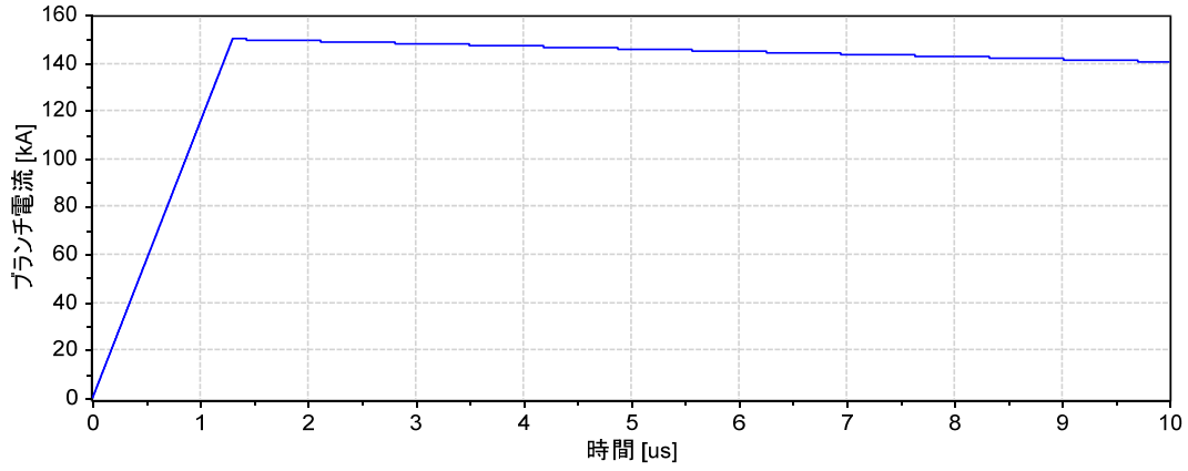
(a) 雷撃電流波形
