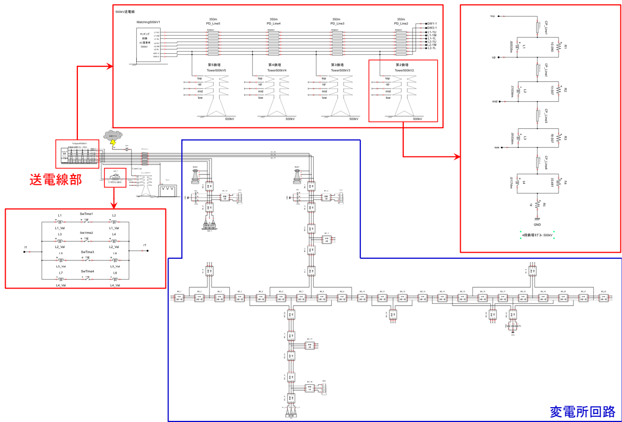
図2 XTAP 入力例
